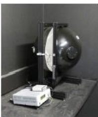
Ulbrichtkugel Vermessung LED
